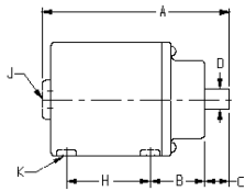
Double Side Lug
