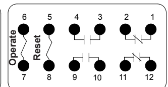
255BXB (2 N.O. + 2 N.C.)
