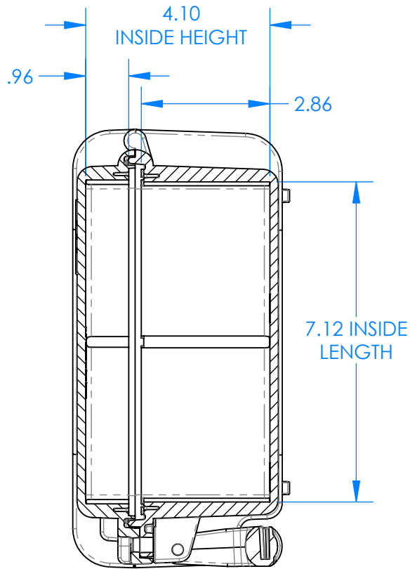
SECTION A-A
