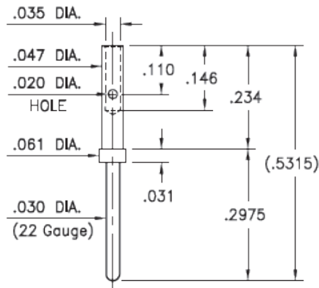
Dimensions per M39029/58-360
