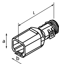
Receptacle 180°
