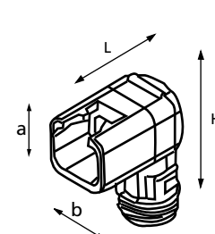
Plug 90°
