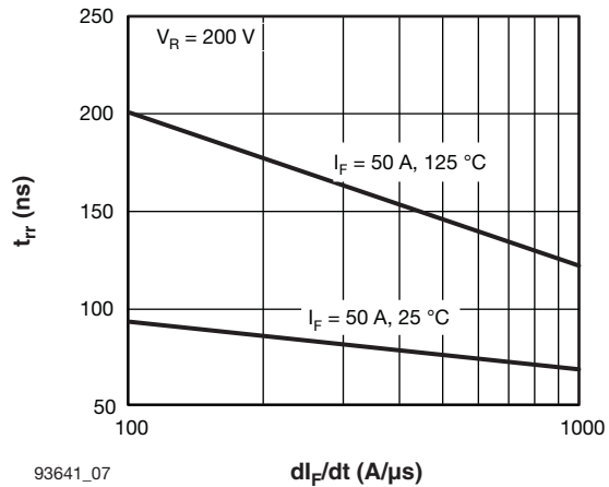
93641_07 di F /dt (A/μs) Fig. 7 - Typical Reverse Recovery Time vs. di F /dt
