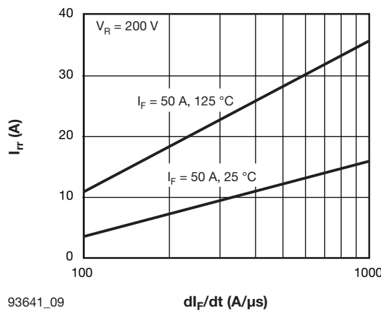
93641_09 di F /dt (A/μs) Fig. 9 - Typical I rr Diode vs. di F /dt
