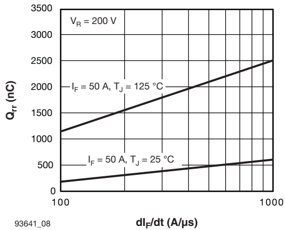
93641_08 di F /dt (A/μs) Fig. 8 - Typical Stored Charge vs. di F /dt
