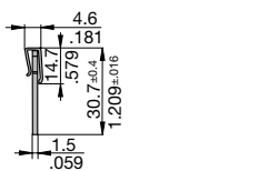
Plug-on cap, 1-pole Y 307 851 01
