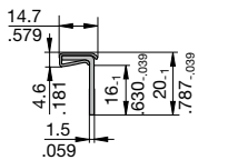
Plug-on cap, 1-pole Y 307 851 01
