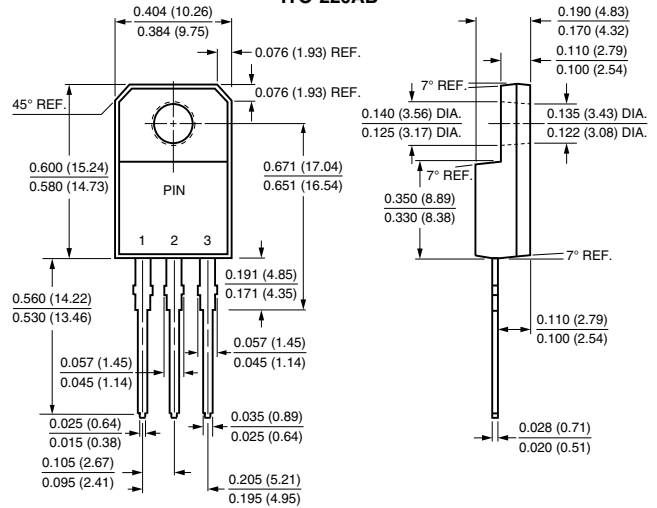
ITO-220AB
