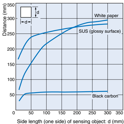
E3Z-D□1(D□6)
