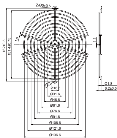
FG-17B For 172mm Fan
