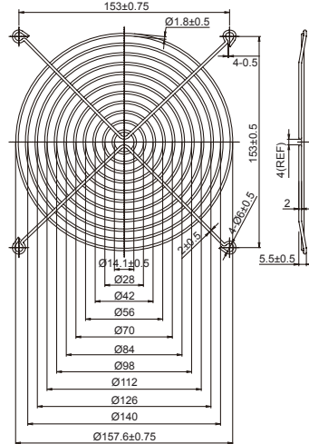
FG-18A For 176mm Fan
