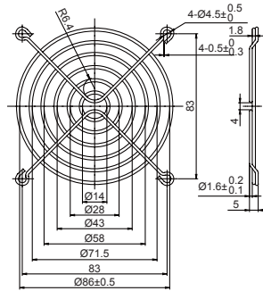
FG-09 For 92mm Fan
