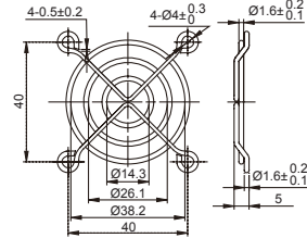
FG-05 For 50mm Fan
