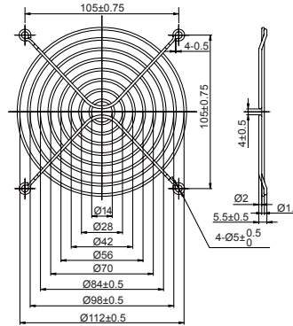
FG-12 For 120mm Fan
