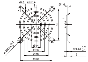
FG-06 For 60mm Fan
