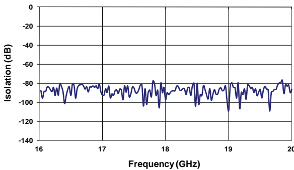
Isolation (16-20 GHz)
