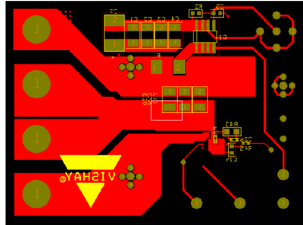
Fig. 11 - Bottom Layer
