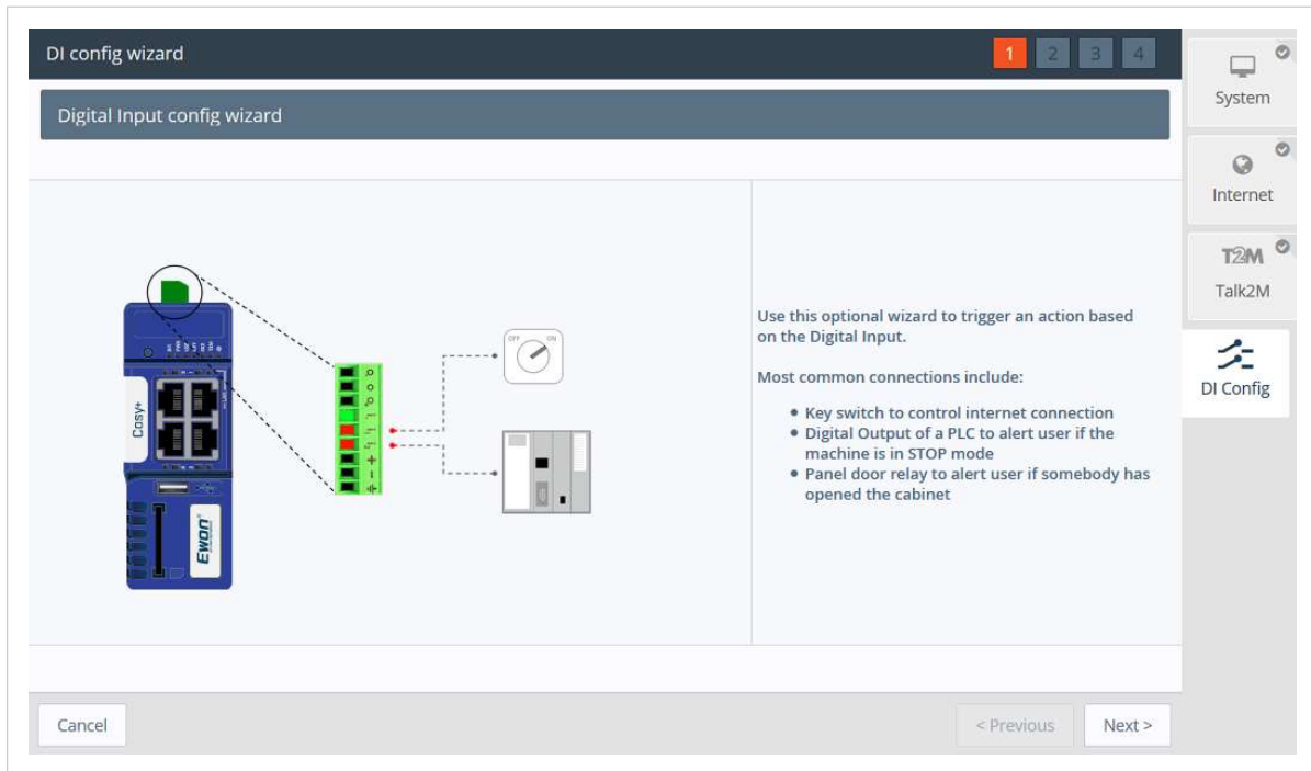
Figure 16. DI Wizard
