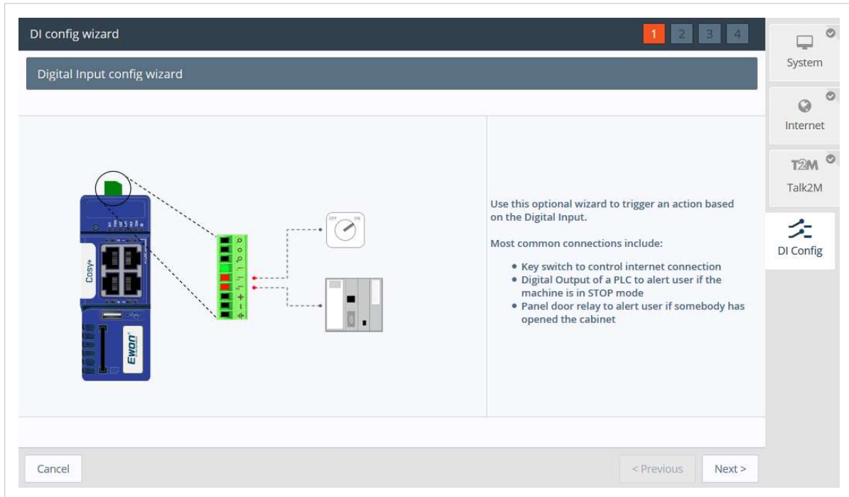
Figure 14. DI Wizard
