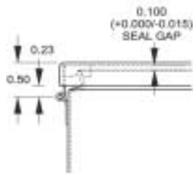
Hinge Side
