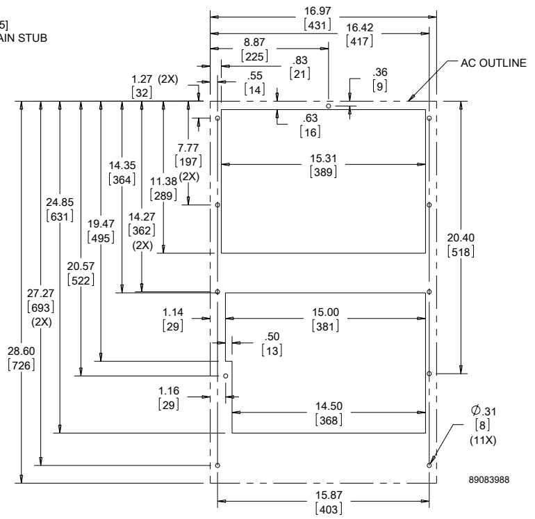
Cutout Dimensions
