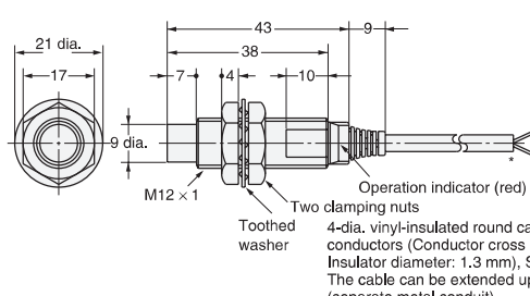
Diagram 8 E2E-X5MY□
