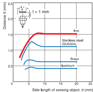
E2E-X10E/-X10Y/-X10F
