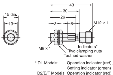
Diagram 16 E2E-X3D□-M1(G) E2E-X2E□-M1/E2E-X2F□-M1
