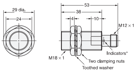
Diagram 20 E2E-X7D□-M1(G)/E2E-X5E□-M1/X5F□-M1 E2E-X5Y□-M1
