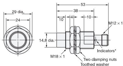
Diagram 21 E2E-X14MD□-M1(G)/E2E-X10ME□-M1 X10MF□-M1 E2E-X10MY□-M1
