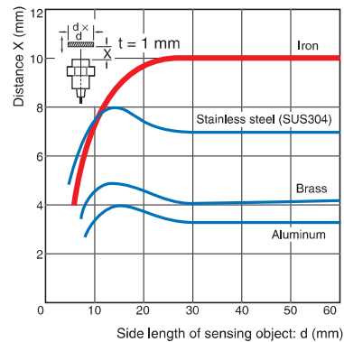
E2E-X10ME/-X10MY/-X10MF
