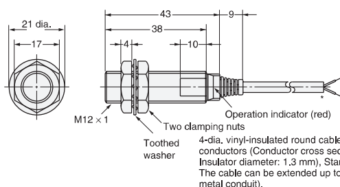
Diagram 7 E2E-X2Y□
