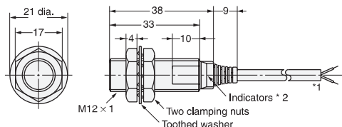
Diagram 5 E2E-X3D□ E2E-X2E□/F□
