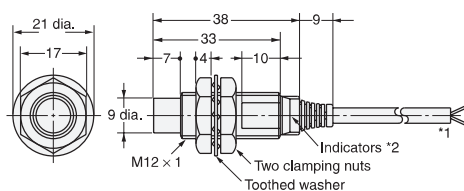
Diagram 6 E2E-X8MD□ E2E-X5ME□/F□
