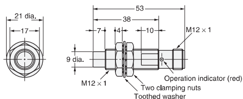
Diagram 19 E2E-X5MY□-M1
