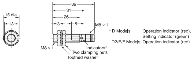
Diagram 24 E2E-X2D□-M3G/E2E-X1R5E□-M3/X1RF□-M3
