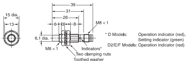
Diagram 25 E2E-X4MD□-M3G/E2E-X2ME□-M3/X2MF□-M3
