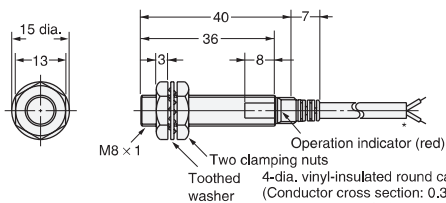
Diagram 3 E2E-X1R5Y□
