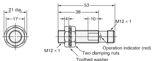
Diagram 18 E2E-X2Y□-M1
