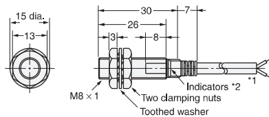
Diagram 1 E2E-X2D□ E2E-X1R5E□/F□
