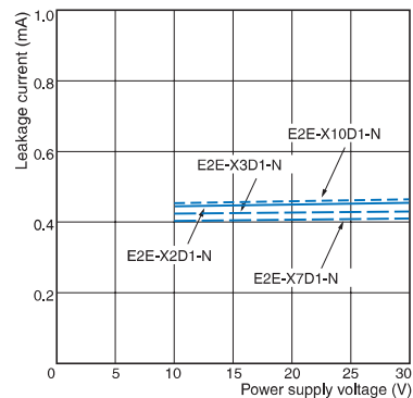
E2E-X□D□
