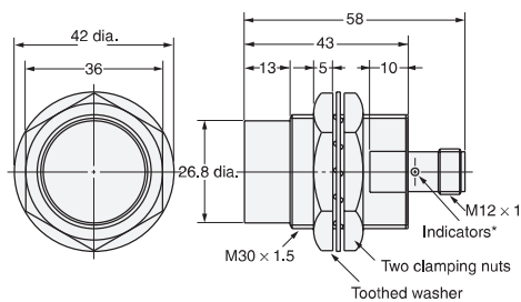
Diagram 23 E2E-X20MD□-M1(G)/E2E-X18ME□-M1/ X18MF□-M1 E2E-X18MY□-M1
