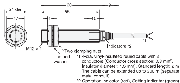
Diagram 10 E2E-X7D□/E2E-X5E□/F□ E2E-X5Y□/E2E-X7T1
