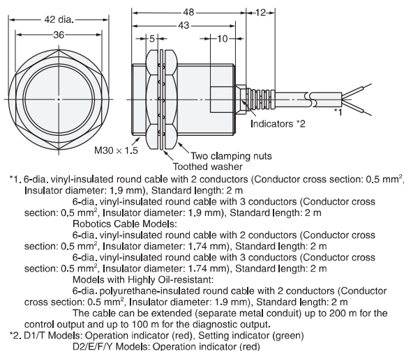
Diagram 12 E2E-X10D□/E2E-X10E□/F□ E2E-X10Y□/E2E-X10T1
