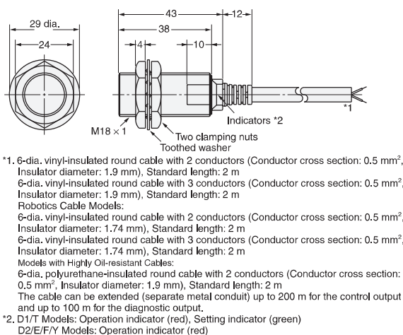
Diagram 12 E2E-X10D□/E2E-X10E□/F□ E2E-X10Y□/E2E-X10T1
