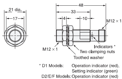
Diagram 18 E2E-X2Y□-M1
