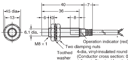
Diagram 4 E2E-X2MY□
