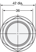
Diagram 33 E2E-X20MD1-M1GJ E2E-X20MD1-M1TGJ E2E-X20MD□-M1TGJ-US
