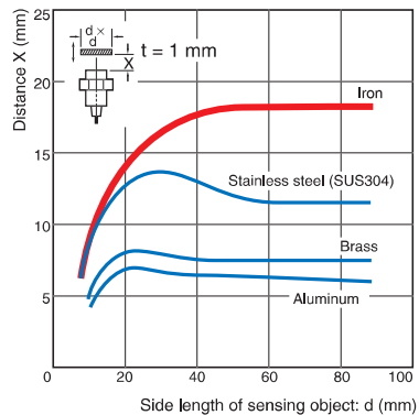
E2E-X18ME/-X18MY/-X18MF
