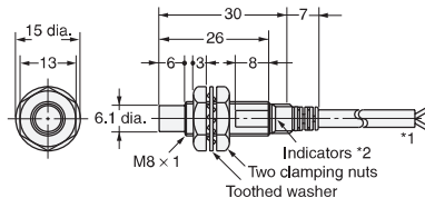
Diagram 2 E2E-X4MD□ E2E-X2ME□/F□
