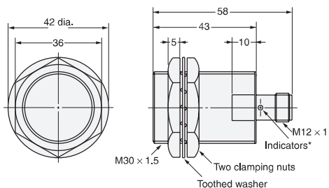
Diagram 22 E2E-X10D□-M1(G)/E2E-X10E□-M1/X10F□-M1 E2E-X10Y□-M1
