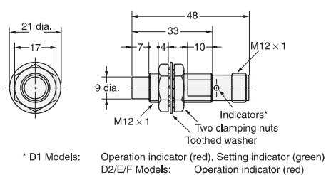
Diagram 19 E2E-X5MY□-M1
