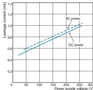
E2E-X□T1
