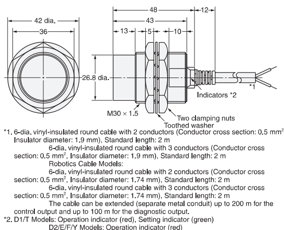
Diagram 13 E2E-X20MD□/E2E-X18ME□/F□ E2E-X18MY□
